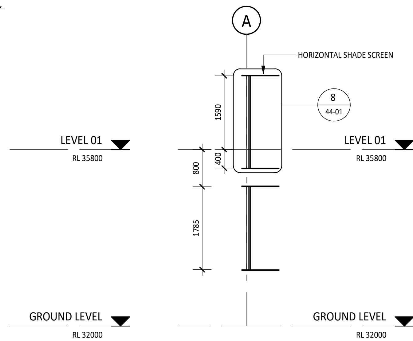
5 SHADE SCREEN SECTION 1 : 50
